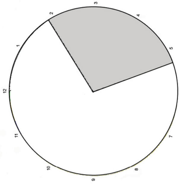
Archaen
