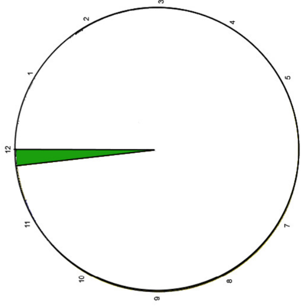
Cenozoic
